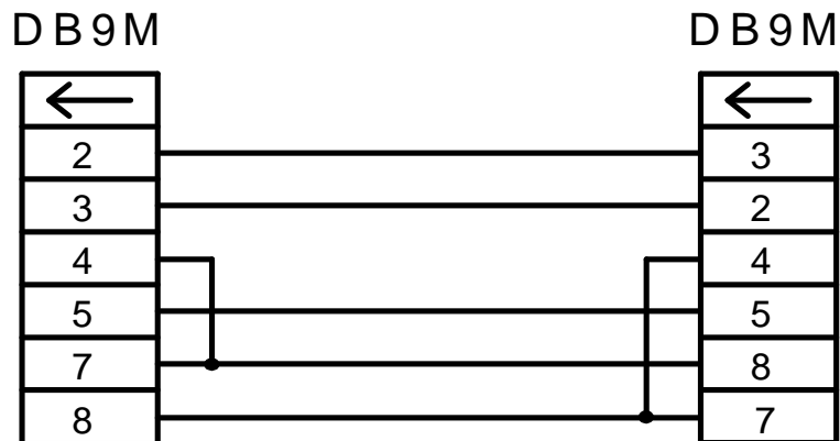
Рисунок 5 – Схема кабелю для підключення до ПР232-01 пристрою переносу інформації CHIP-USB.
