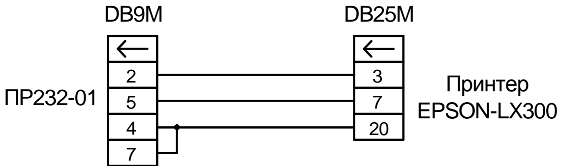
Рисунок 4 – Схема кабелю для підключення до ПР232-01 принтера EPSON-LX300.
