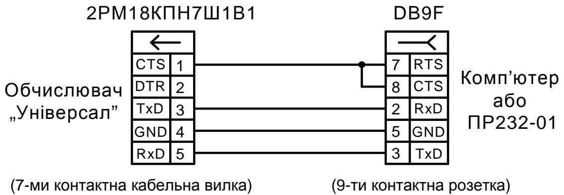
Рисунок 2 – Схема кабелю для підключення до ПР232-01 обчислювача „Універсал” випуску до 2004 року, який не проходив модернізації.
