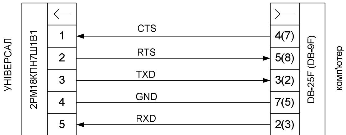
Рис. 2 Схема розпайки комунікаційного кабелю з інтерфейсом RS-232
