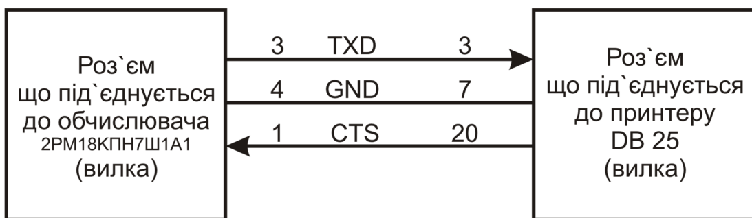
Рис. 5 Схема розпайки кабелю для з'єднання обчислювача і принтера
